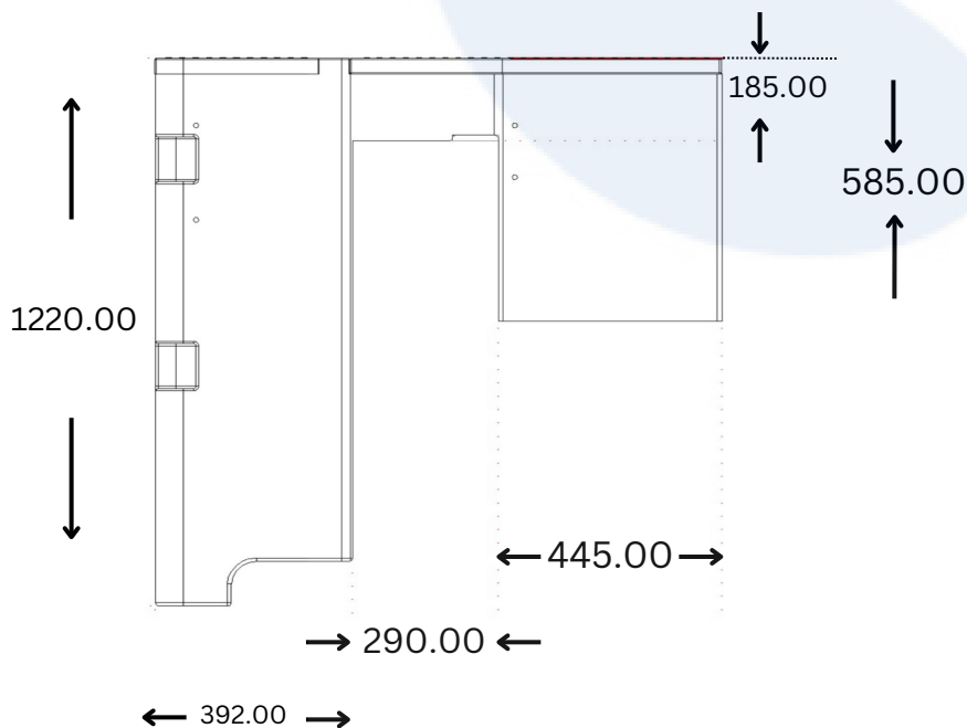
side elev.
